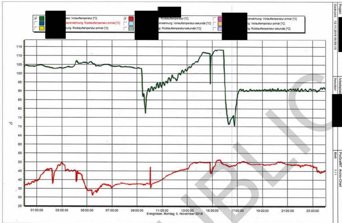
Temperaturverlauf Fernwärmeversorgung
